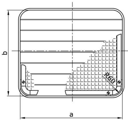
Жалюзи без щитка
