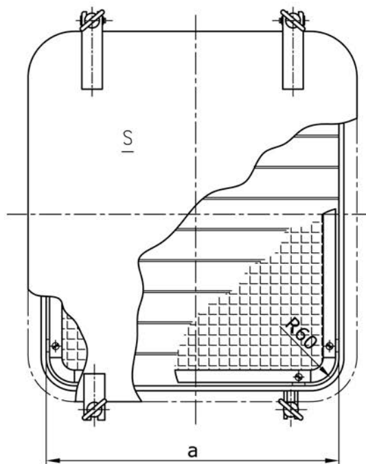
Жалюзи со щитком
